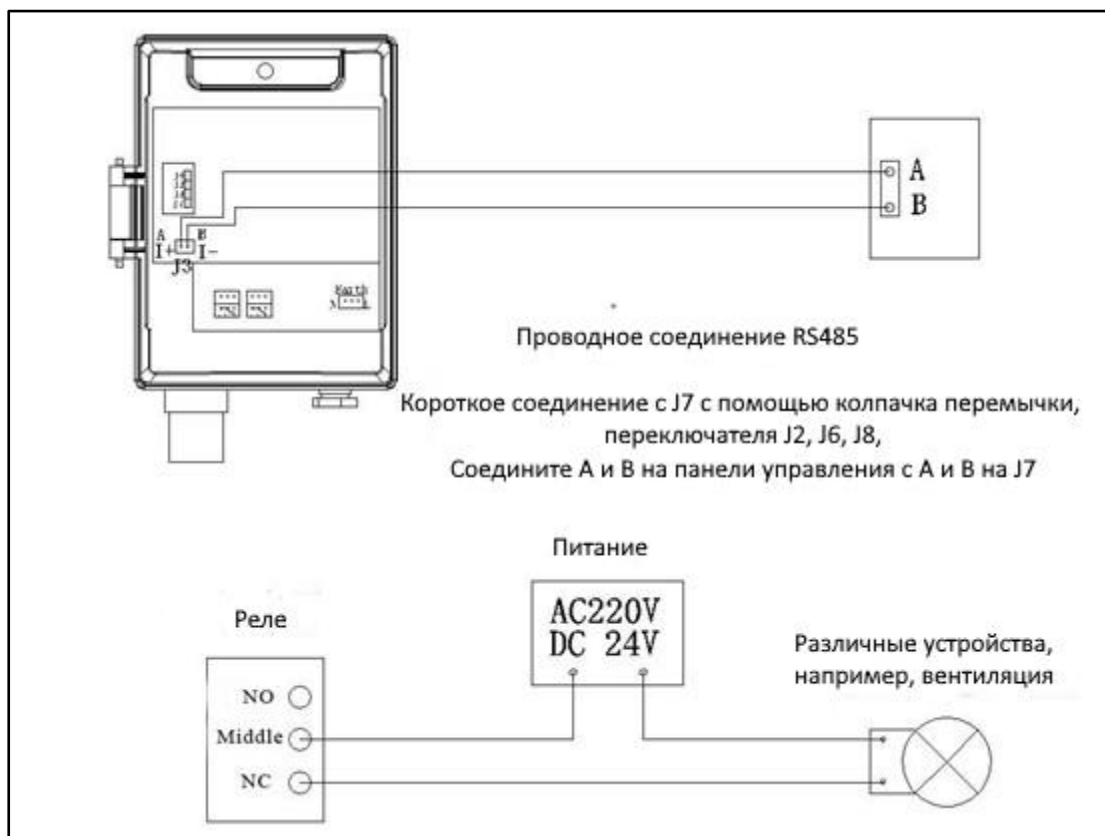
Рис. 3.2 Проводное соединение RS485
